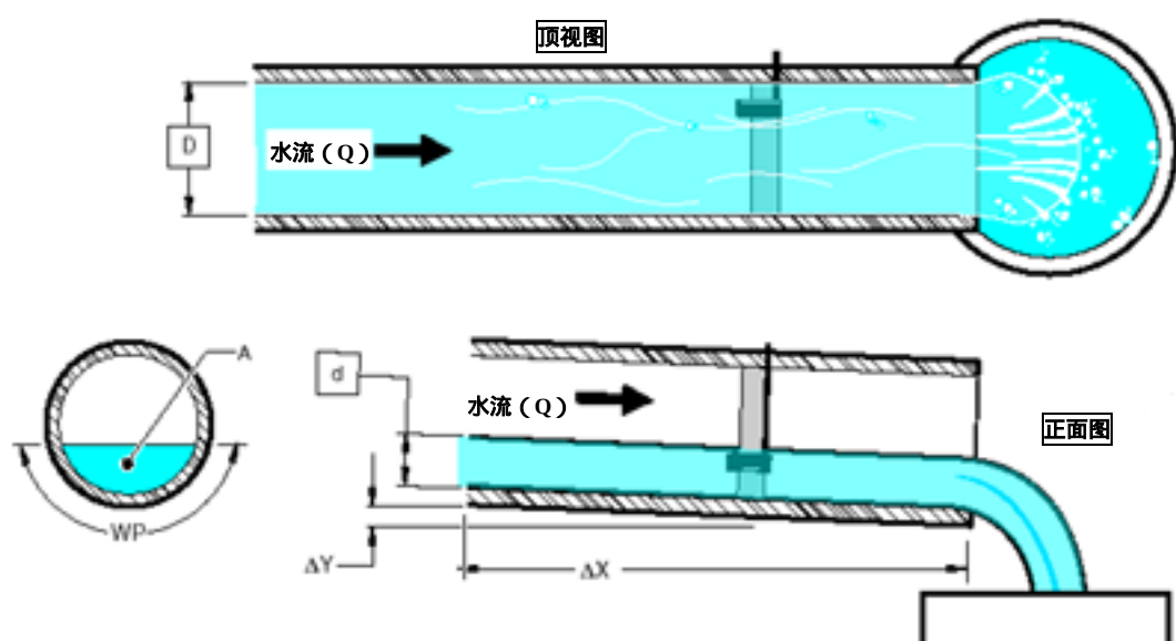
图 55 圆形管道
